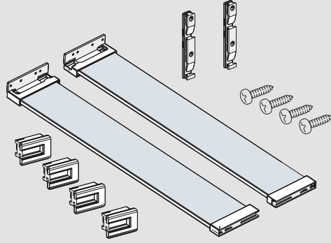
Parçalar / Parts
